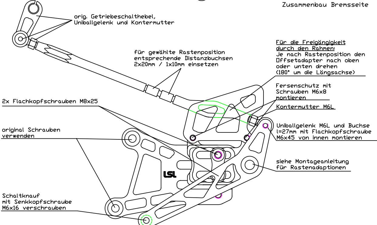
Rastenanlage Yamaha YZF-R1 '04- Zusammenbau Bremsseite
